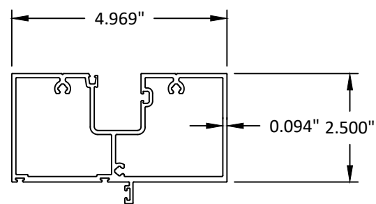
55 DOOR HEAD
