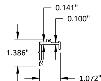
11 FLUSH FILLER
